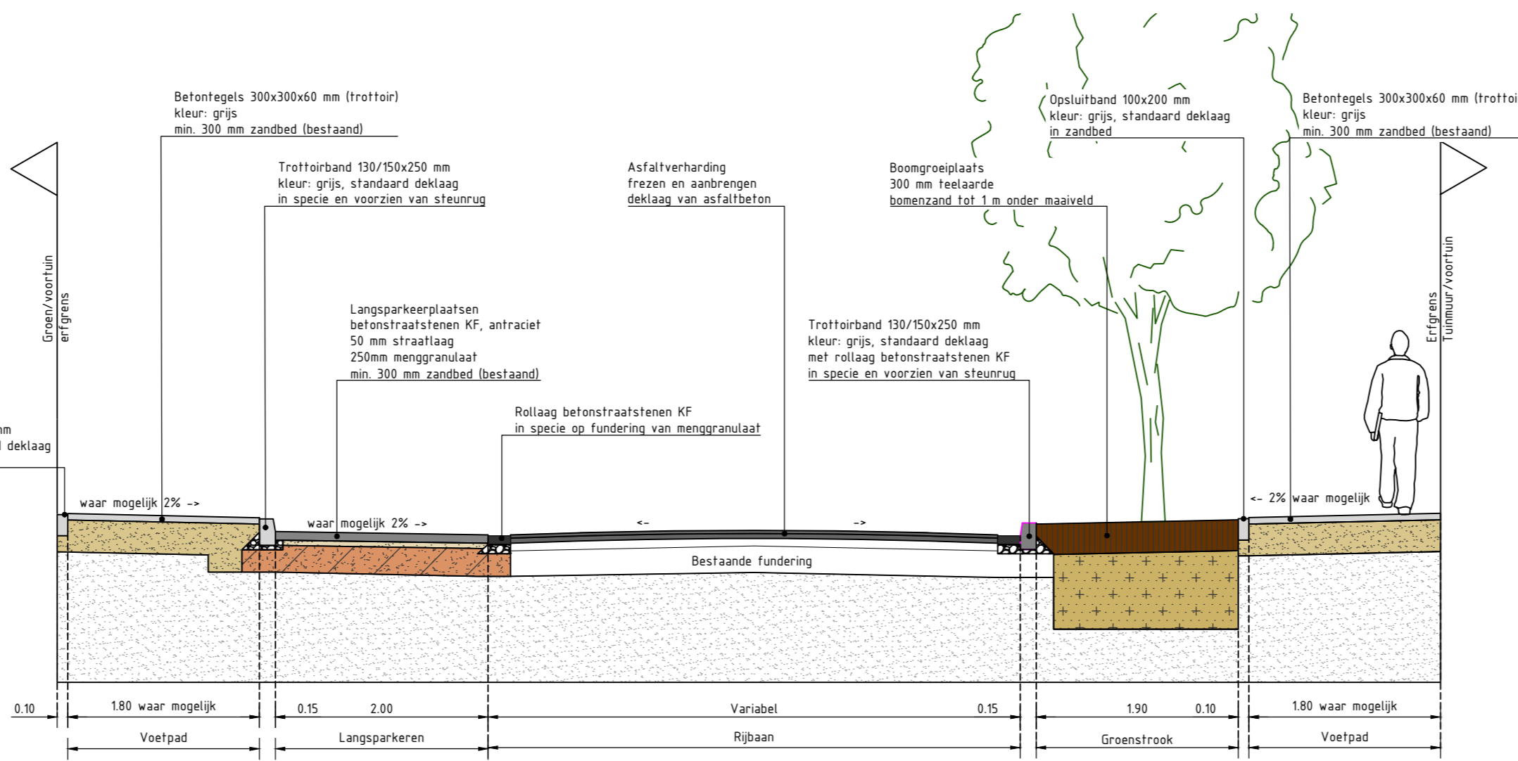
Principe profiel Principe rollaag met trottoir en groeiplaats schaal 1:50
