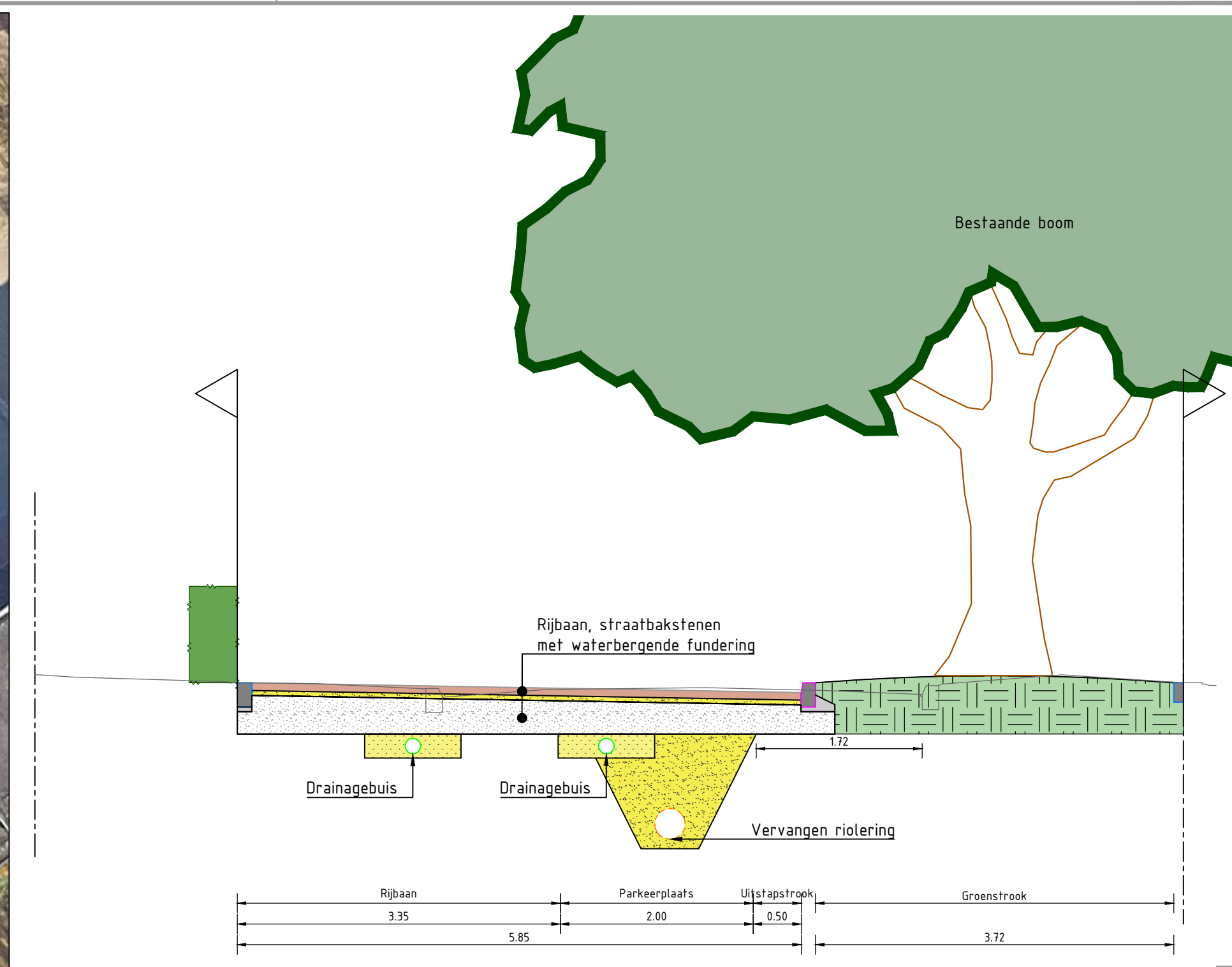
Doorsnede A-A Schaal 1:50
